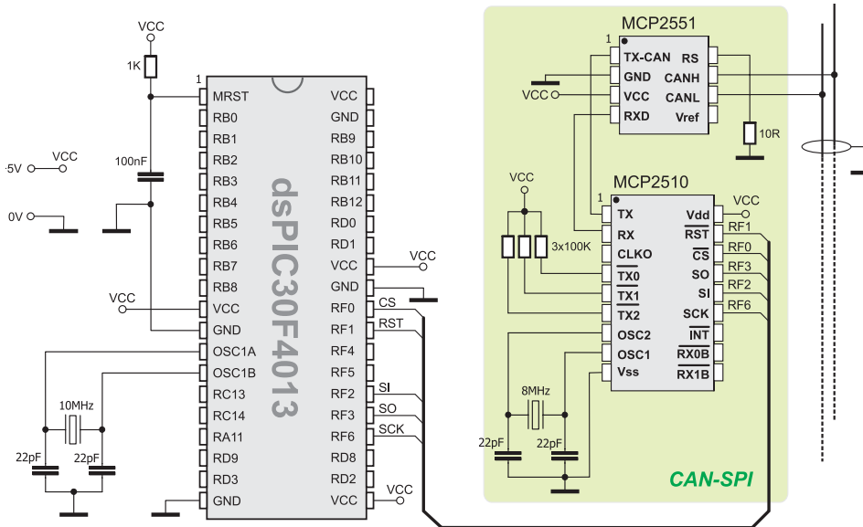
Šema 1. Povezivanje CAN-SPI modula sa dsPIC30F4013 mikrokontrolerom
