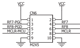
dsPICprog CONNECTOR
